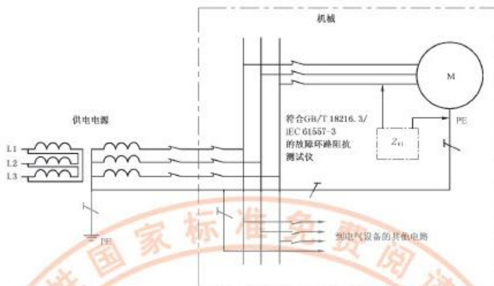
图 A.1 故障环路阻抗测量典型配置
